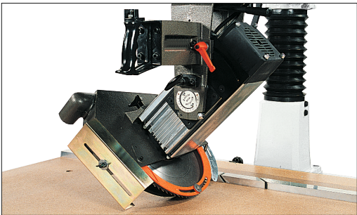
Carrello a 8 cuscinetti con guide intercambiabili
