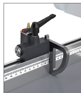
Referencia lateral neumática de 60 mm (opcional).
