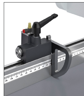
Référence latérale pneumatique 60 mm. (en option)
