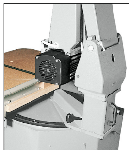
Bâti du pendule orientable
